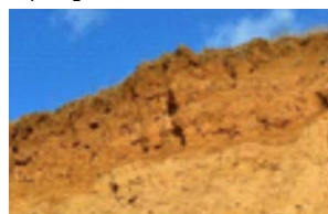
Д) элювий
