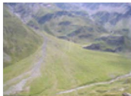
Б) пролювий
